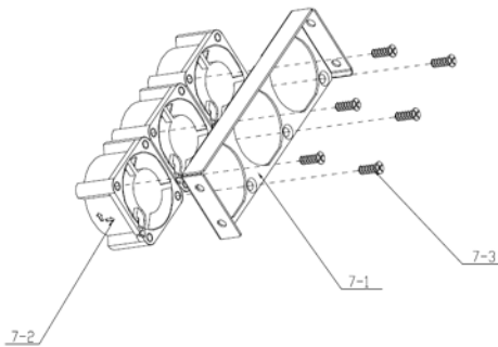
Figure 5 Remove the Fan from Fan rack
